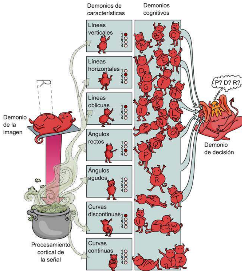
Identificación de un carácter en base al pandemonium. Fuente: Peter H. Lindsay; Donald A. Norman (1983). Introducción a la Psicología Cognitiva (ed. original 1977). Madrid: Tecnos.
